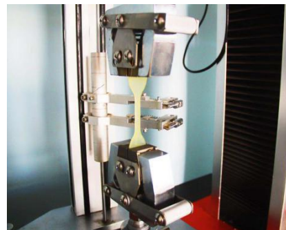
Tensile Test
